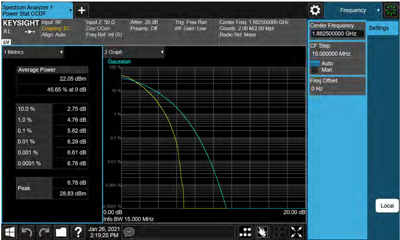
Sub6 n25. PAR Plot (15M BW Ch.376500 64QAM RB 79_0)
