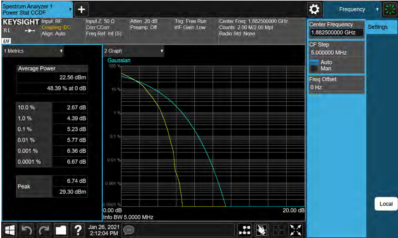
Sub6 n25. PAR Plot (5M BW Ch.376500 16QAM RB 25_0)
