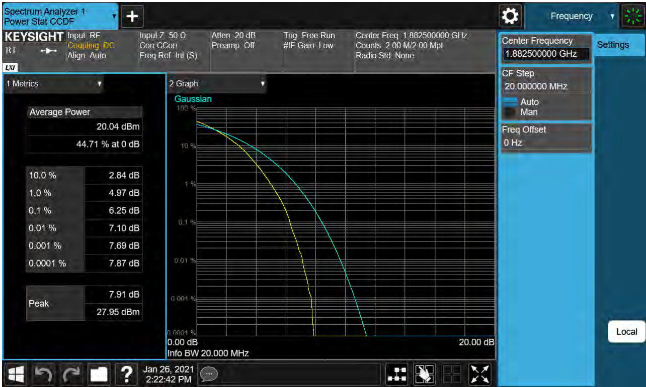
Sub6 n25. PAR Plot (20M BW Ch.376500 256QAM RB 106_0)
