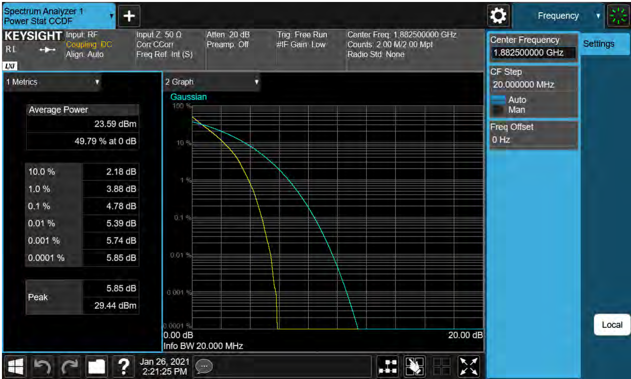
Sub6 n25. PAR Plot (20M BW Ch.376500 QPSK RB 106_0)
