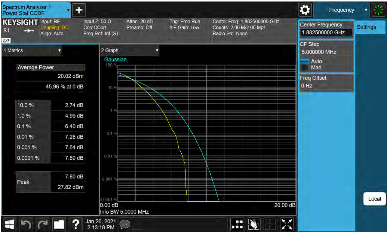
Sub6 n25. PAR Plot (5M BW Ch.376500 256QAM RB 25_0)
