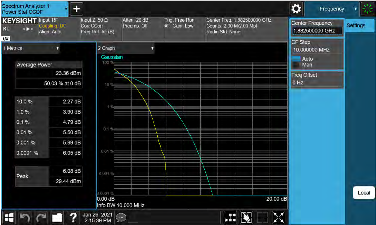
Sub6 n25. PAR Plot (10M BW Ch.376500 QPSK RB 52_0)
