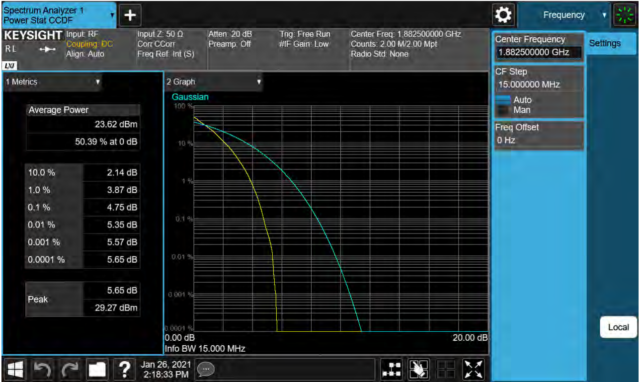
Sub6 n25. PAR Plot (15M BW Ch.376500 QPSK RB 79_0)
