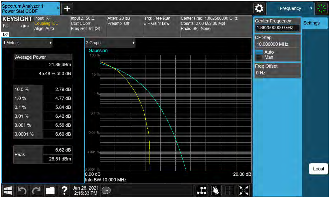
Sub6 n25. PAR Plot (10M BW Ch.376500 64QAM RB 52_0)
