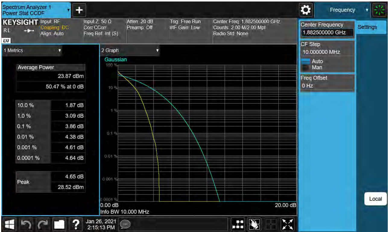
Sub6 n25. PAR Plot (10M BW Ch.376500 BPSK RB 52_0)
