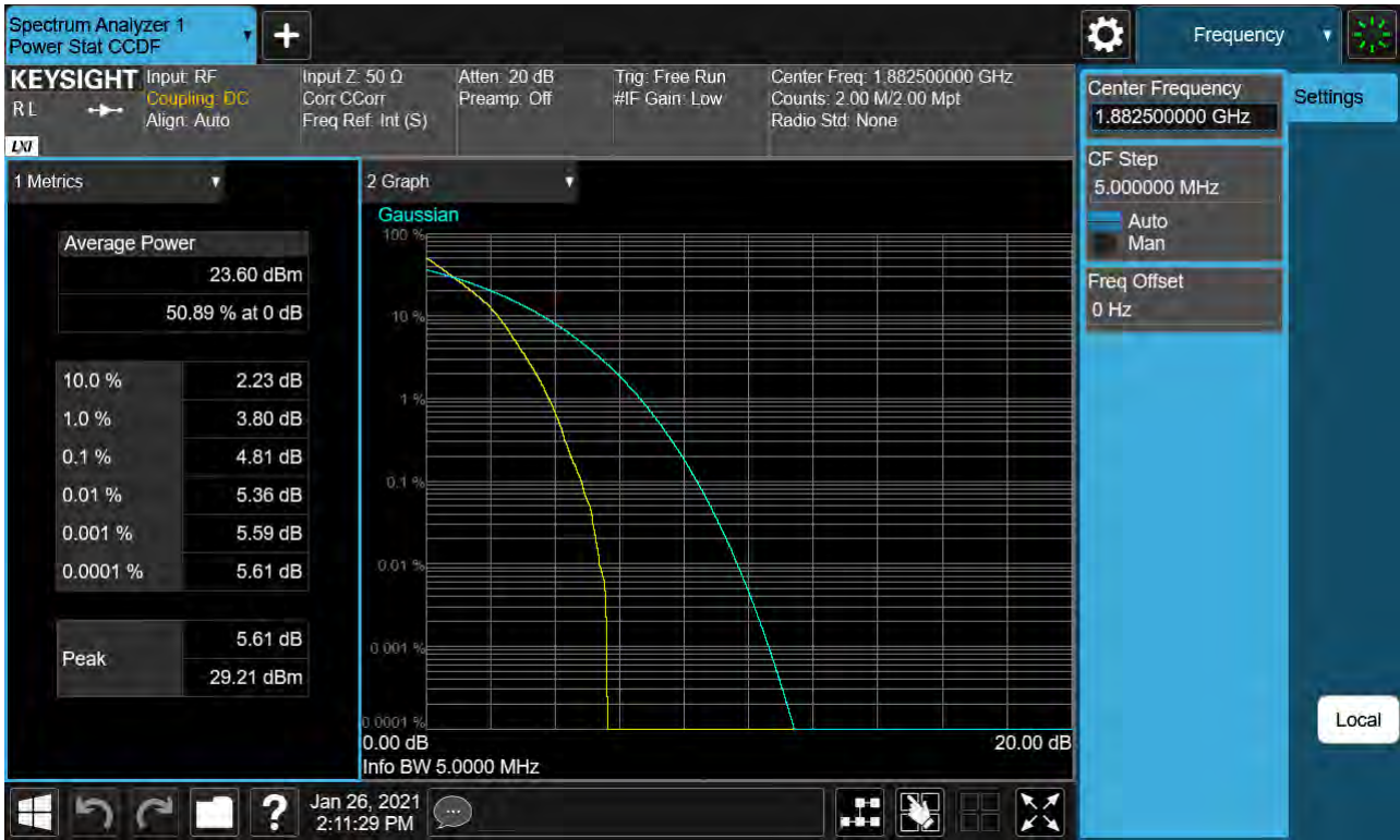
Sub6 n25. PAR Plot (5M BW Ch.376500 QPSK RB 25_0)
