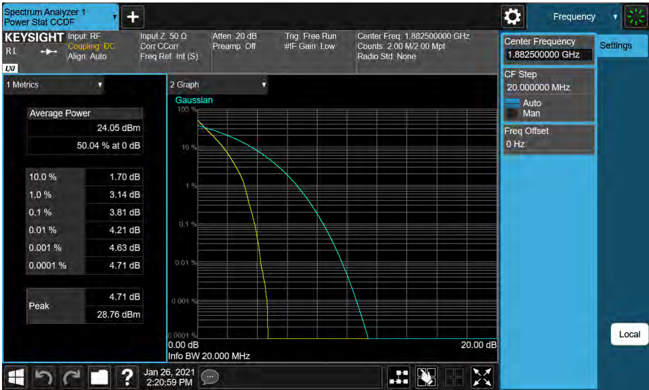
Sub6 n25. PAR Plot (20M BW Ch.376500 BPSK RB 106_0)
