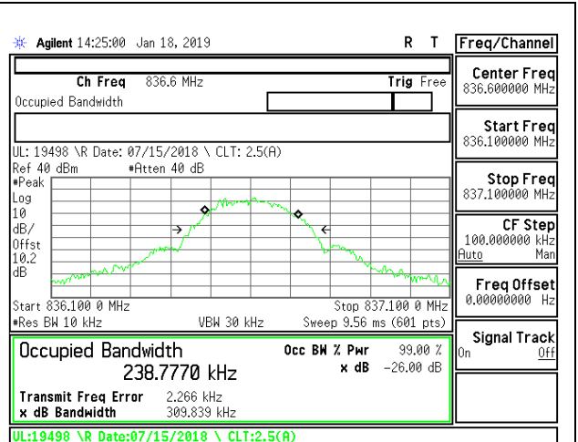
GSM 850MHz EGPRS MID Channel
