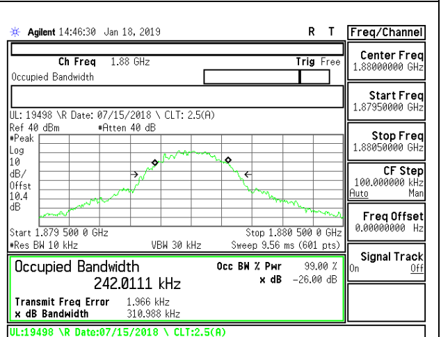
GSM 1900MHz EGPRS MID Channel
