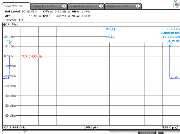
DH5
