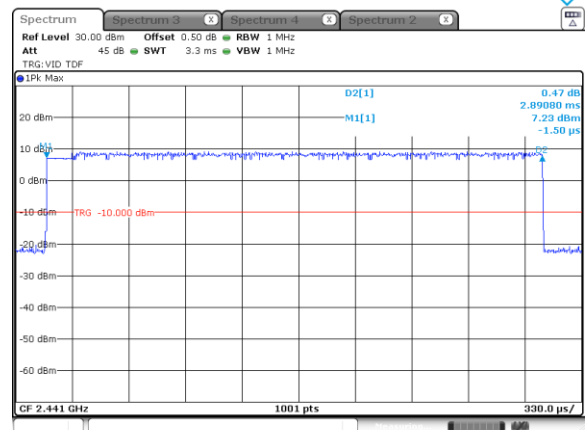
2-DH5
