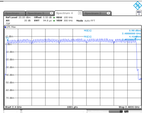
\pi/4 DQPSK
