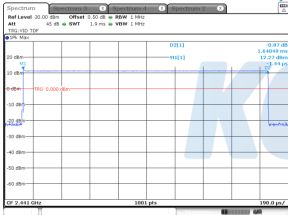
DH3
