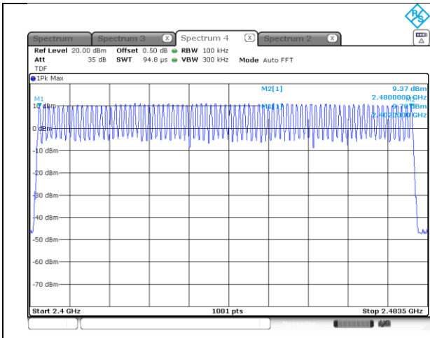
GFSK
