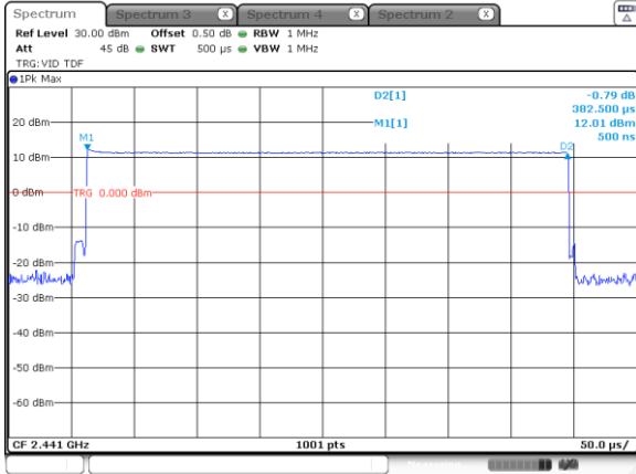
DH1
