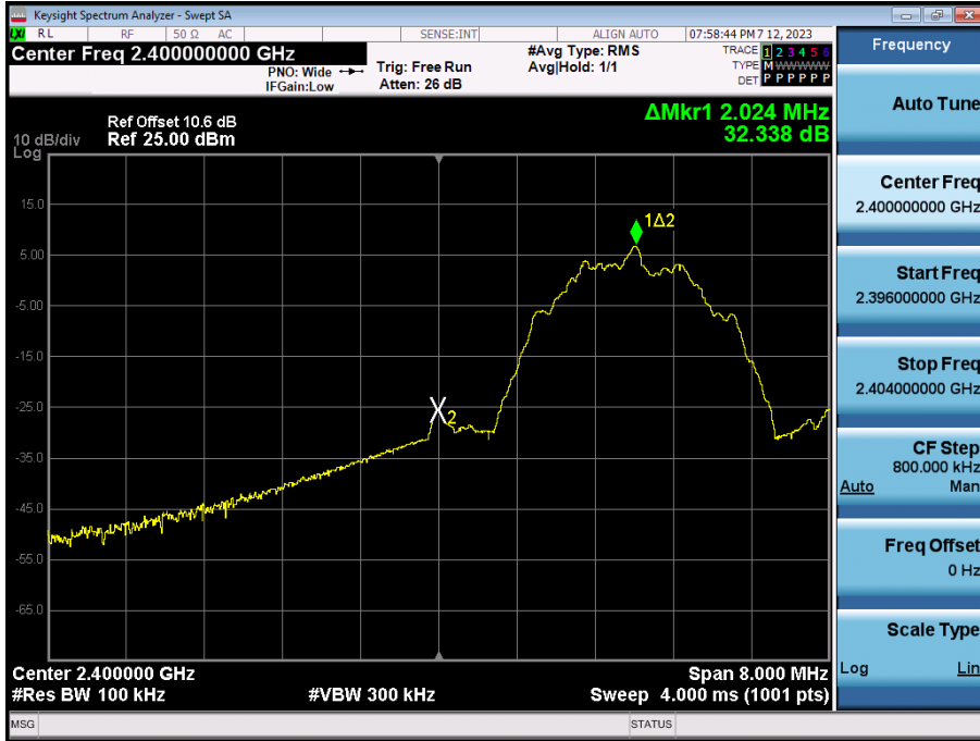
Lower(2M Bit/s 37 Byte)
