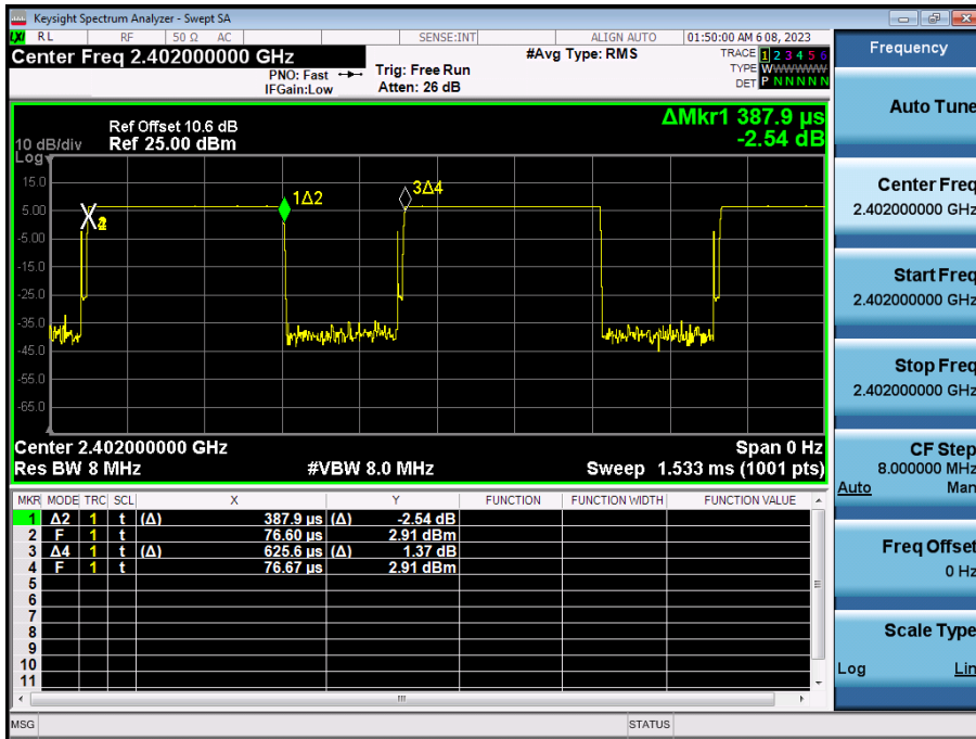
1 M Bit/s (37 Byte)
