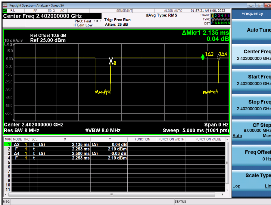
1 M Bit/s (255 Byte)
