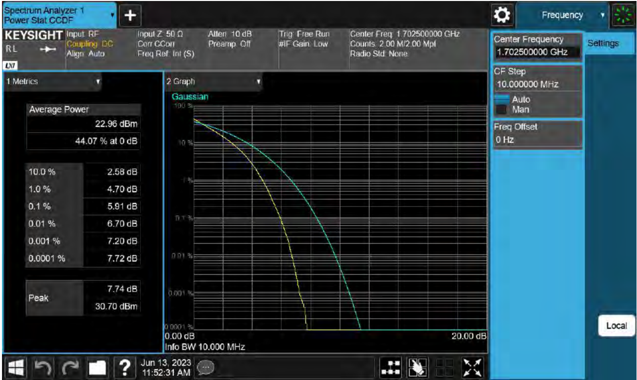
Sub6 n70. PAR Plot (10 M BW_Ch.340500_QPSK_Full RB)
