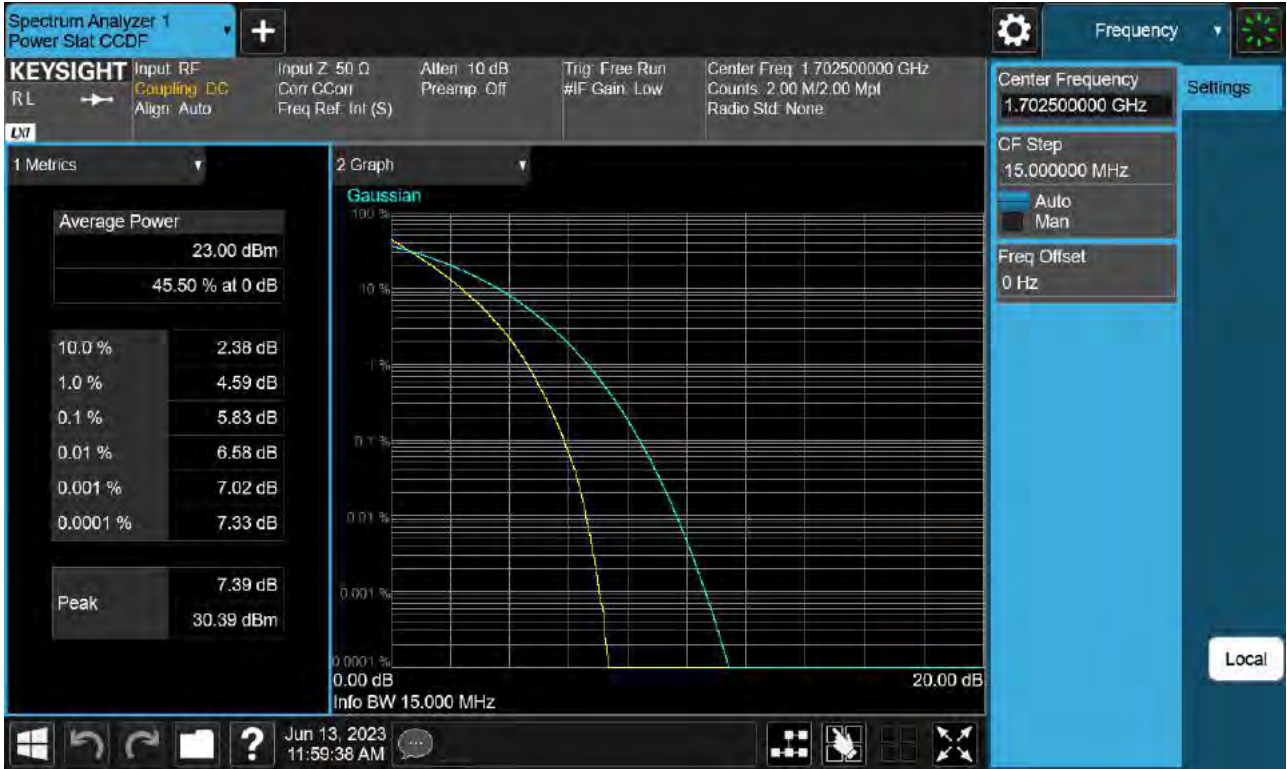
Sub6 n70. PAR Plot (15 M BW_Ch.340500_QPSK_Full RB)
