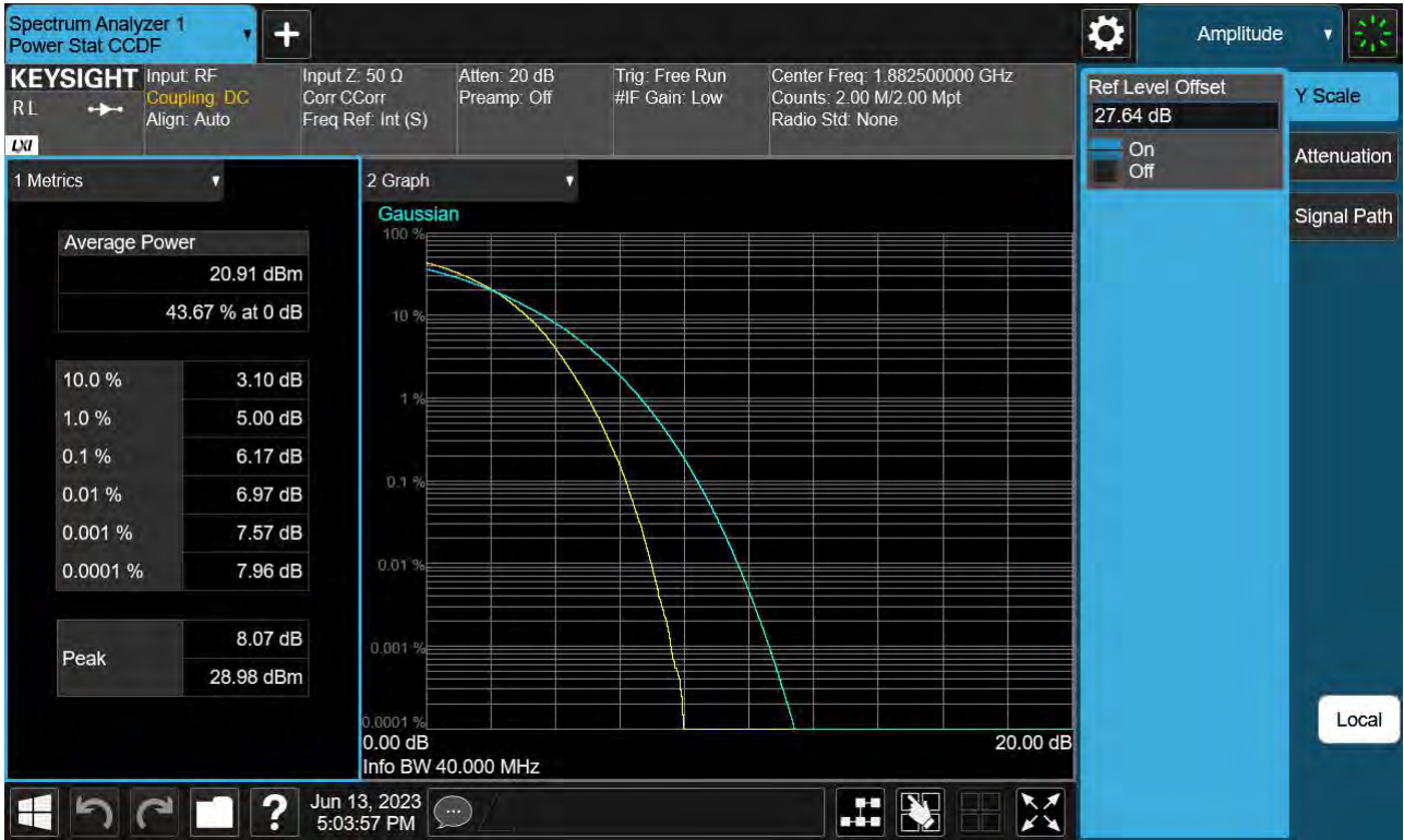
Sub6 n25(2). PAR Plot (40 M BW Ch.376500 64QAM_ Full RB_0)
