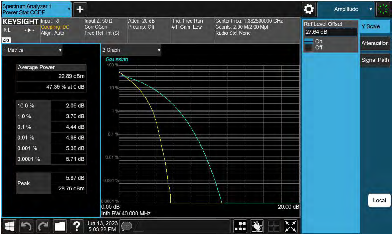
Sub6 n25(2). PAR Plot (40 M BW Ch.376500 BPSK_ Full RB_0 )
