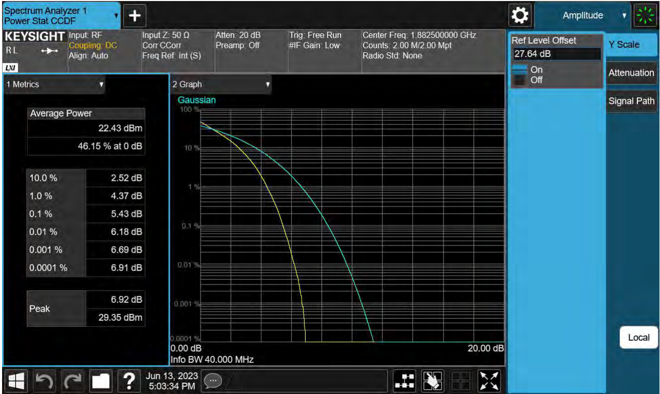
Sub6 n25(2). PAR Plot (40 M BW Ch.376500 QPSK_ Full RB_0 )
