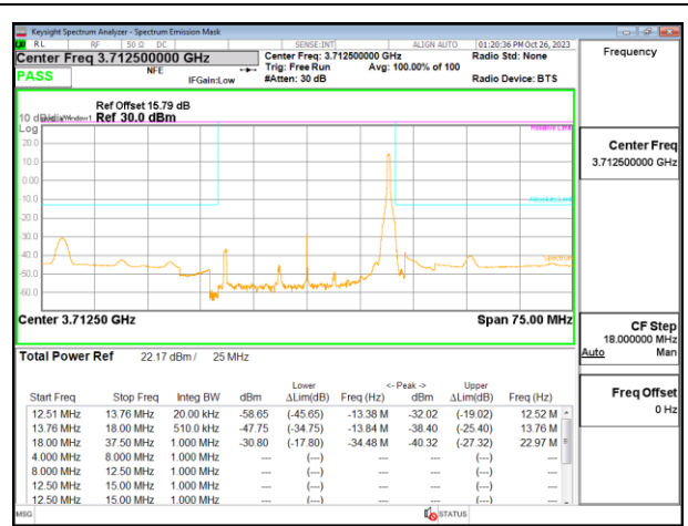
5G NR n77 25MHz QPSK Low Channel RB1-64
