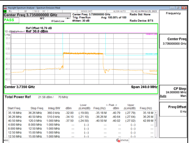
5G NR n77 70MHz QPSK Low Channel RB180-0
