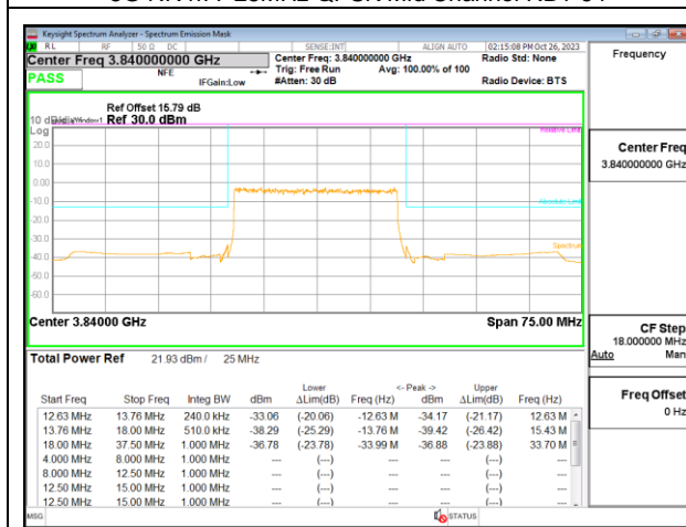
5G NR n77 25MHz QPSK Mid Channel RB64-0
