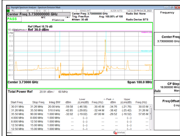
5G NR n77 60MHz QPSK Low Channel RB1-161
