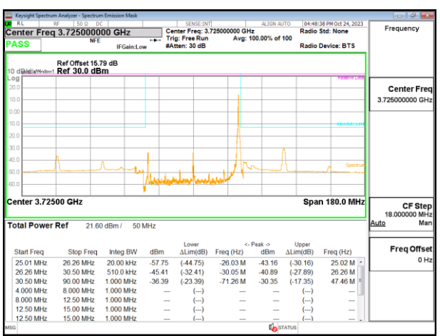
5G NR n77 50MHz QPSK Low Channel RB1-132
