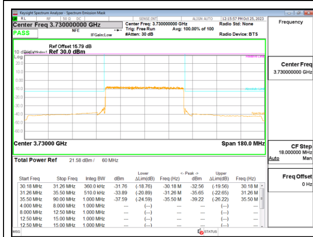
5G NR n77 60MHz QPSK Low Channel RB162-0
