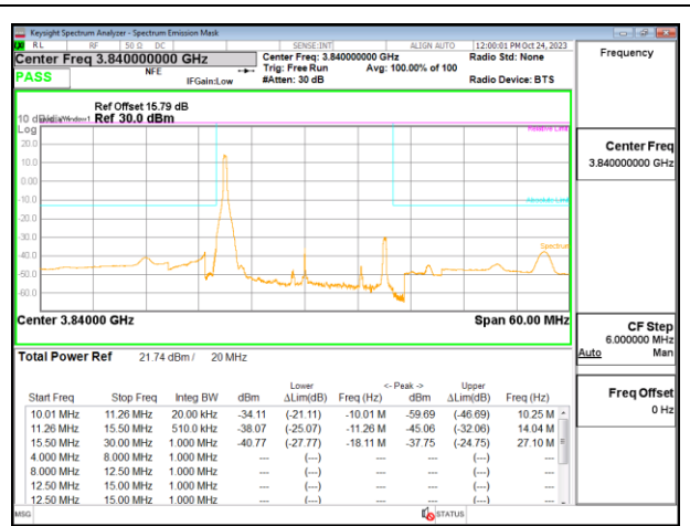
5G NR n77 20MHz QPSK Middle Channel RB1-0:
