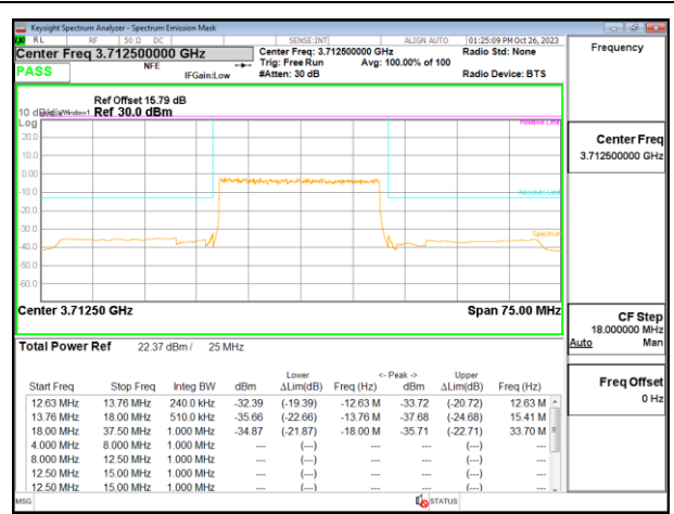
5G NR n77 25MHz QPSK Low Channel RB64-0
