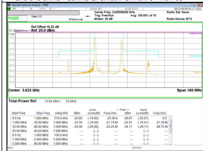
LTE B48 5MHz + 20MHz QPSK Mid Ch RB1-0 + RB1-99
