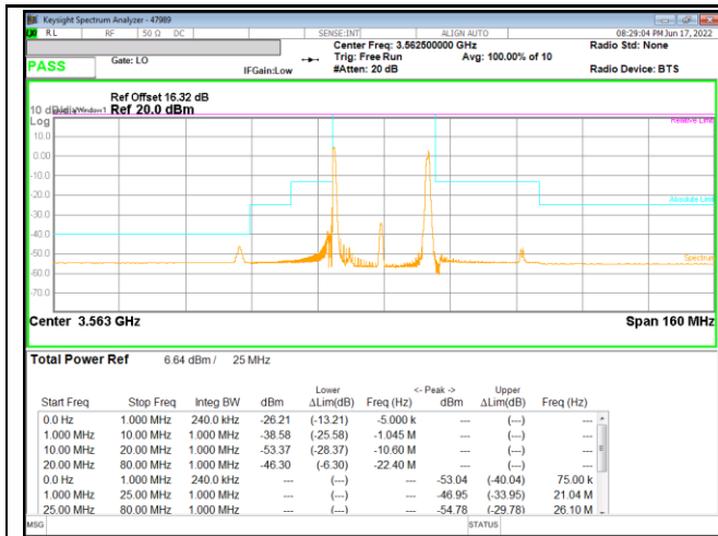
LTE B48 5MHz + 20MHz QPSK Low Ch RB1-0 + RB1-99
