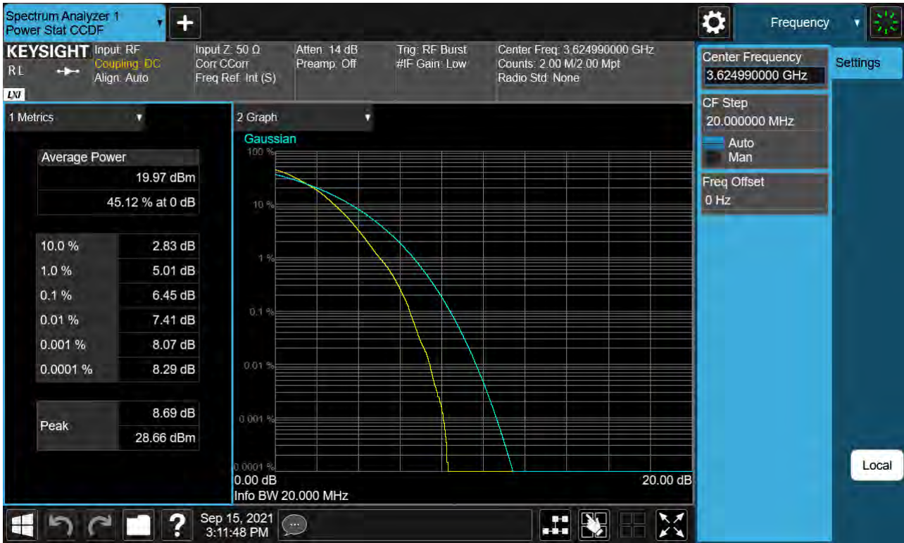
Sub6 n48. PAR Plot (20 MHz Ch.641666 64-QAM RB 50)
