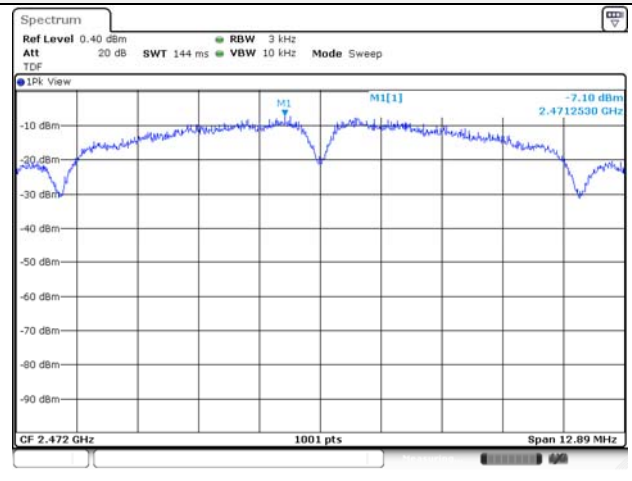
802.11b / 2 472 MHz
