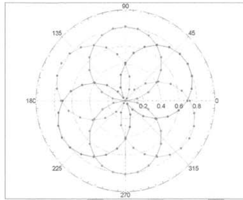
f=1800 MHz,R22
