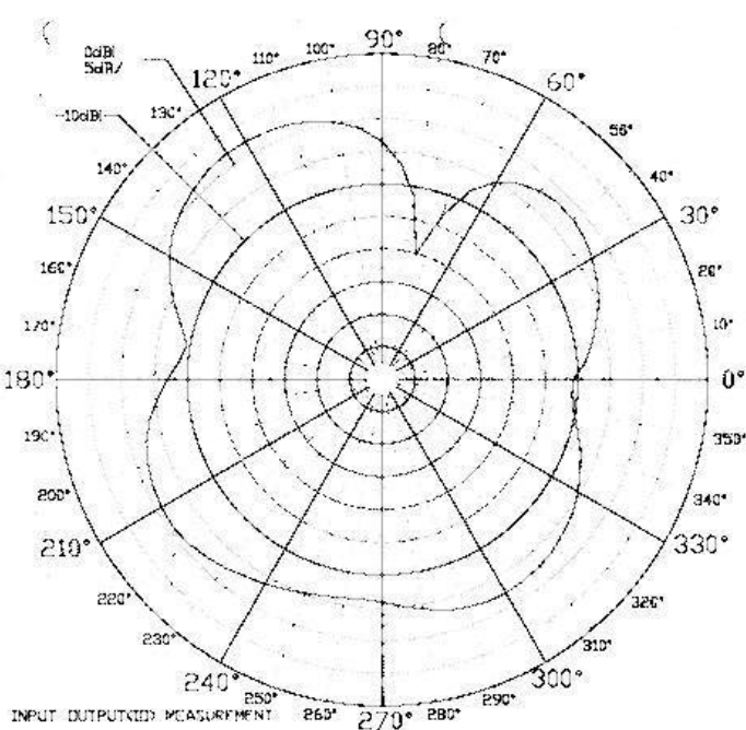
E-Plane
