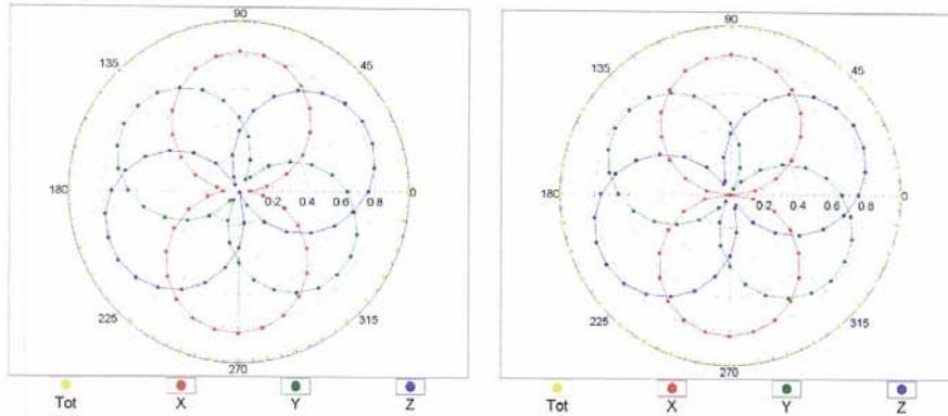
f=1800 MHz,R22
