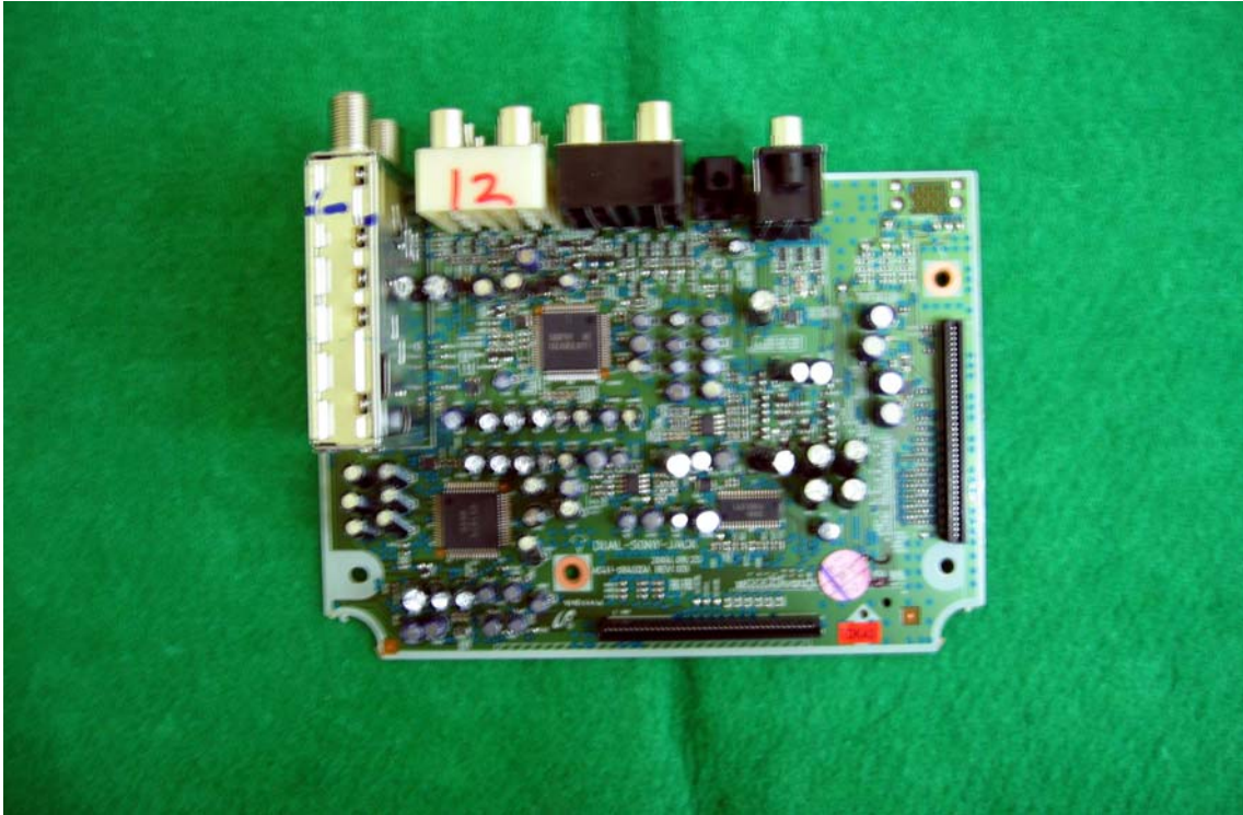
AV PCB View (Top)
