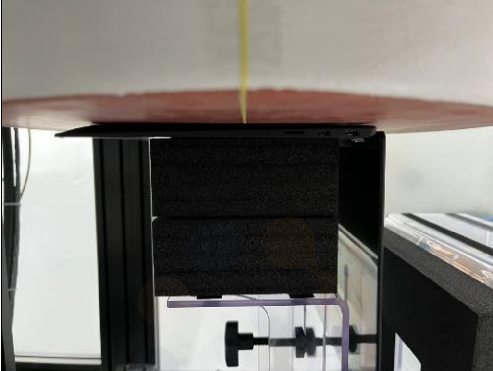
F.1.1) Notebook Mode_Body_Rear (0 mm)
