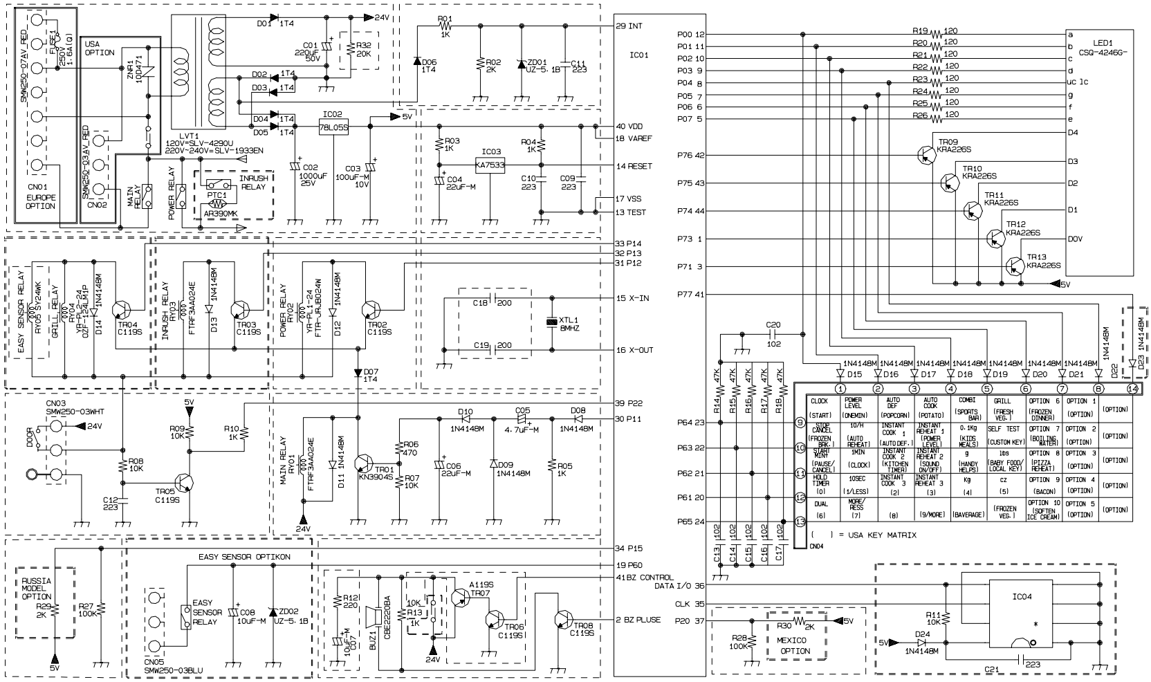
N2LED1 SCHEMATIC
