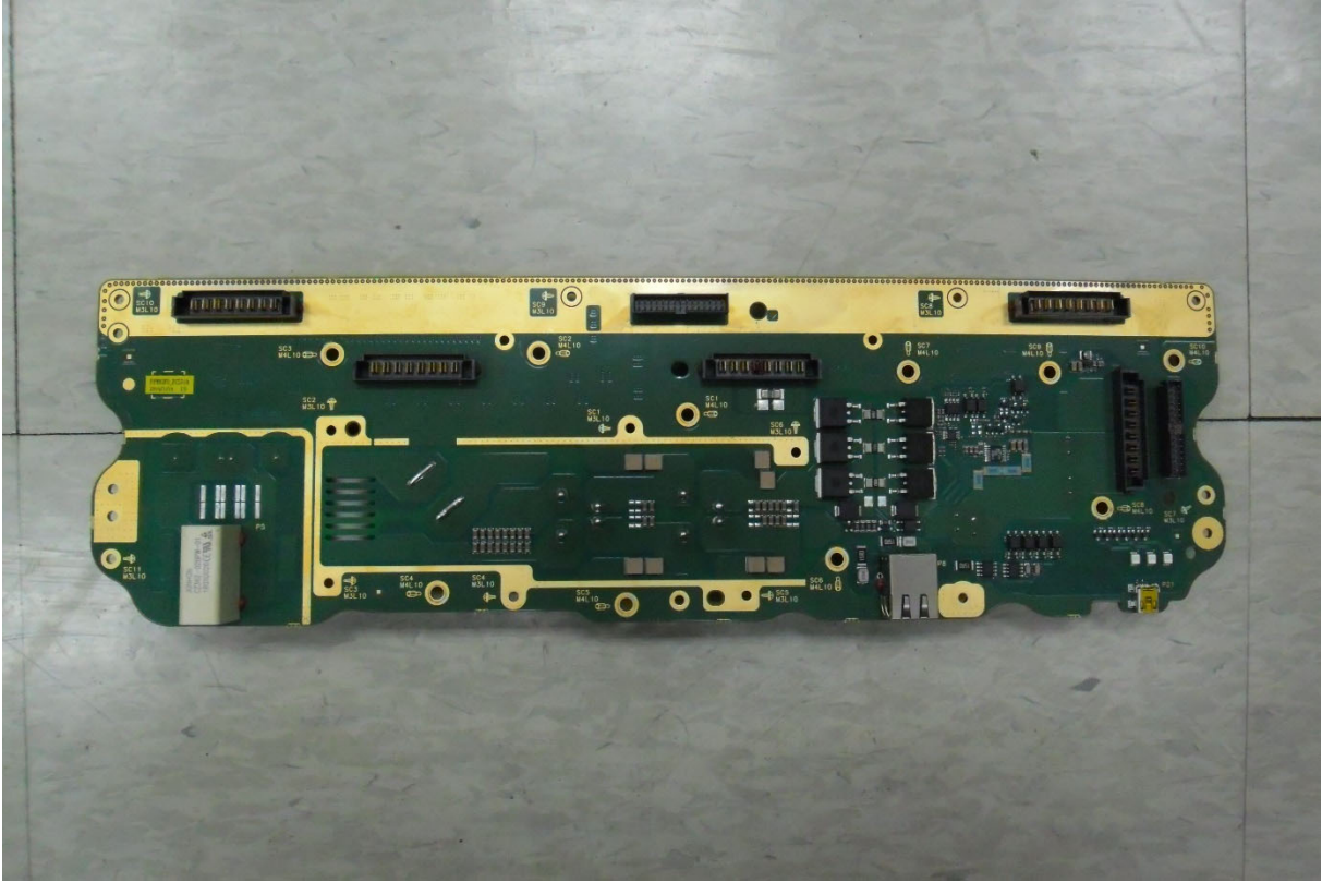
PPWB3F0 Module (Bottom)
