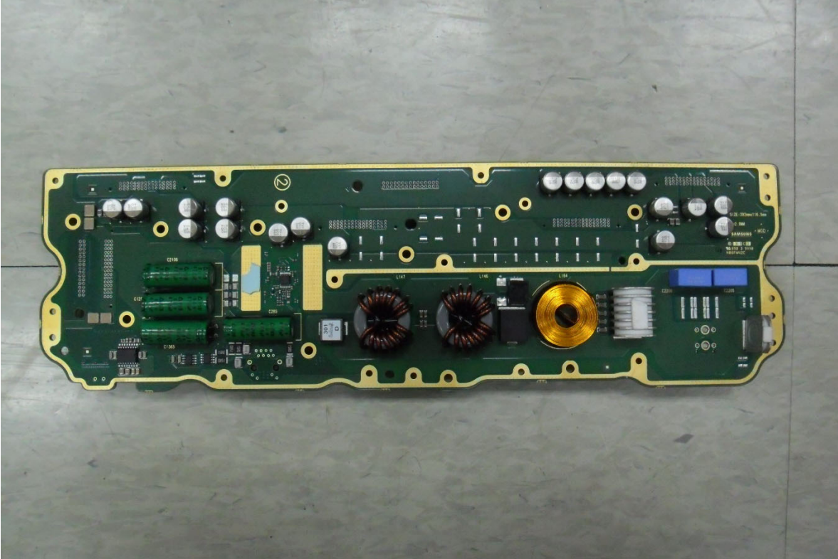
PPWB3F0 Module (Top)
