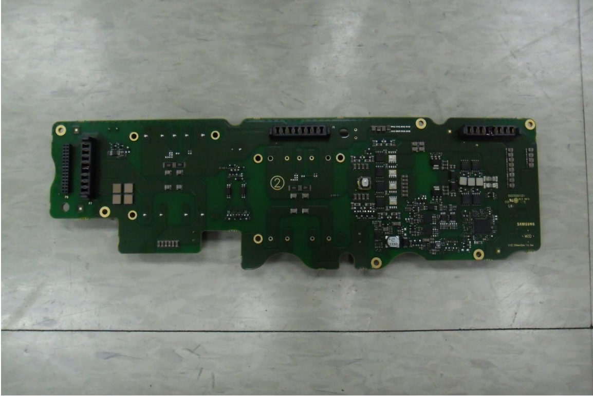
PPWB3F1 Module (Bottom)
