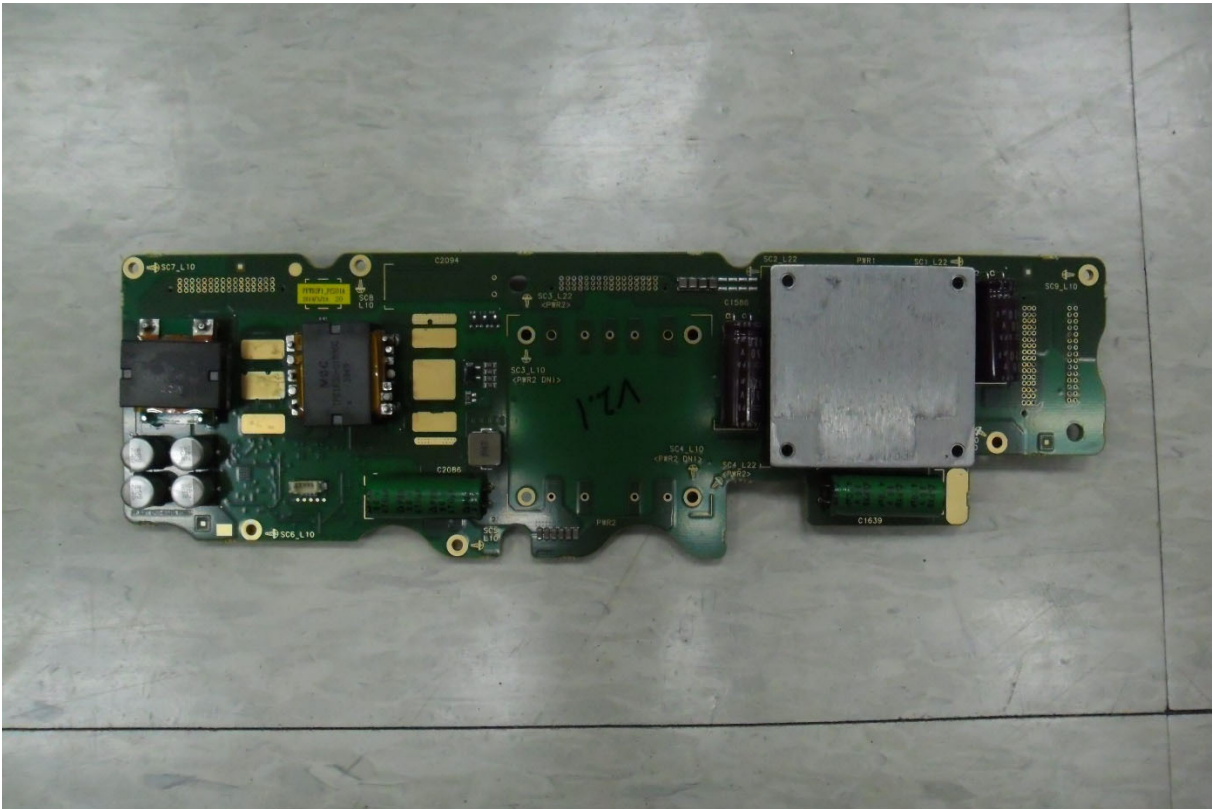
PPWB3F1 Module (Top)
