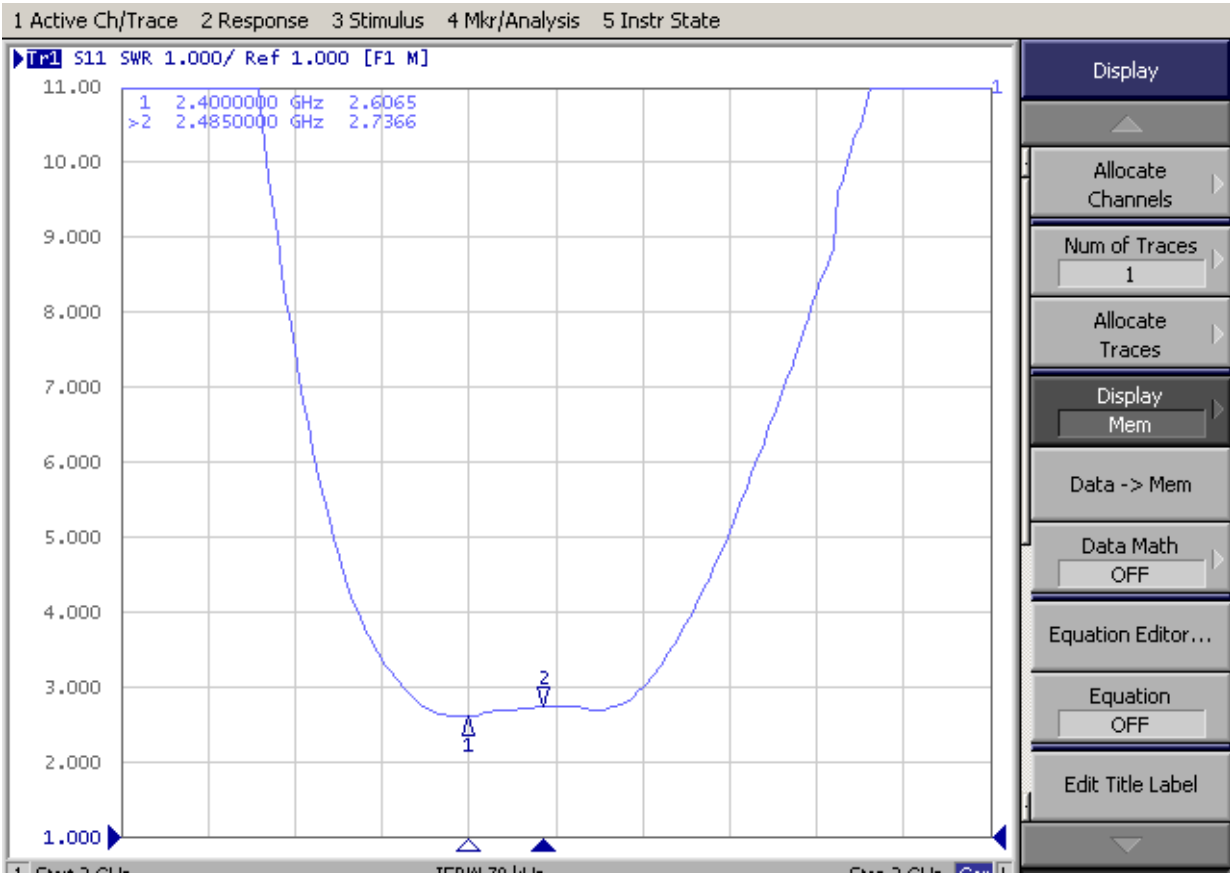
VSWR
