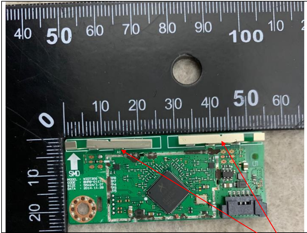
PIFA Antenna
