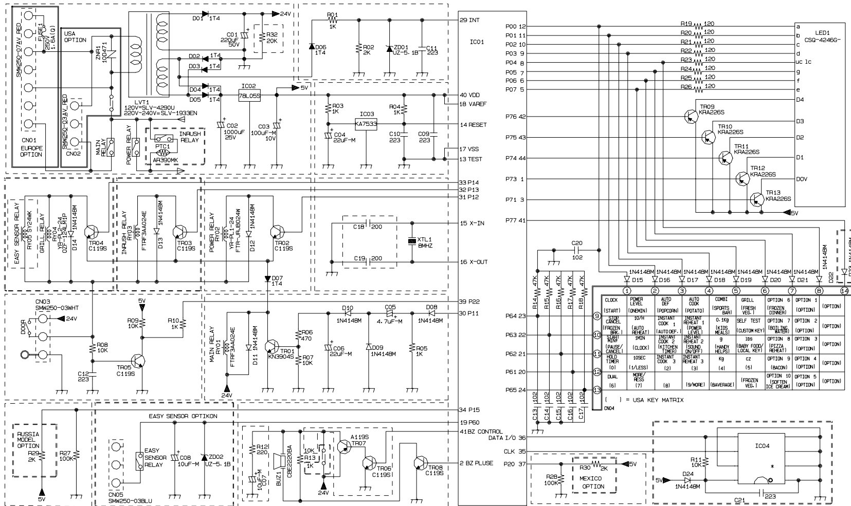
N2LED1 SCHEMATIC
