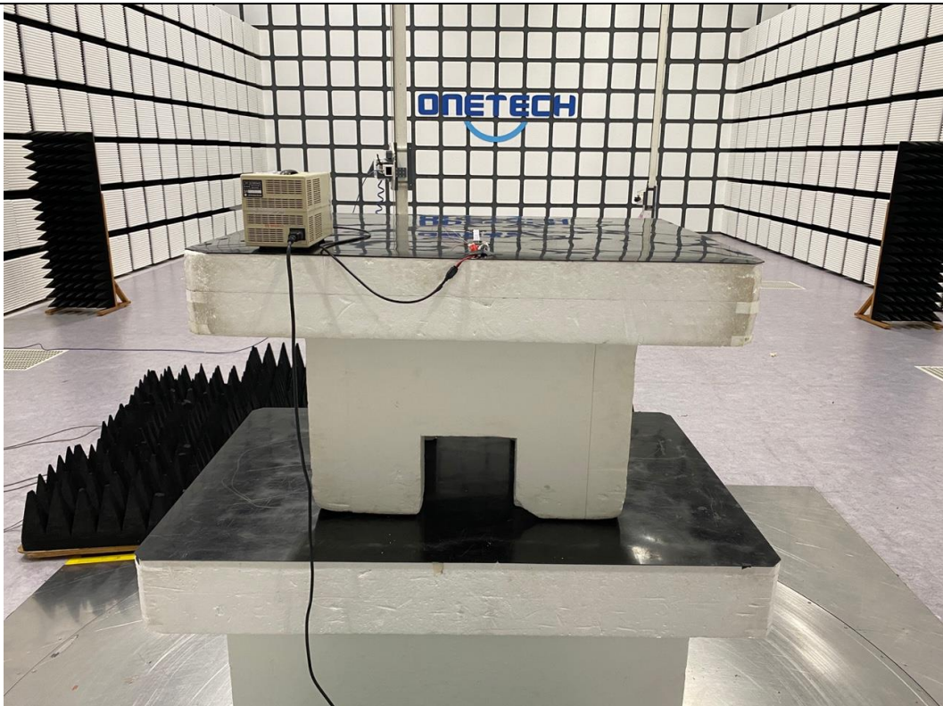
18 GHz ~ 40 GHz
