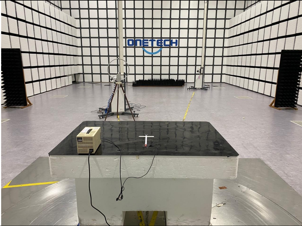
9 kHz ~ 30 MHz
