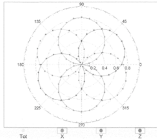
f=1800 MHz,R22
