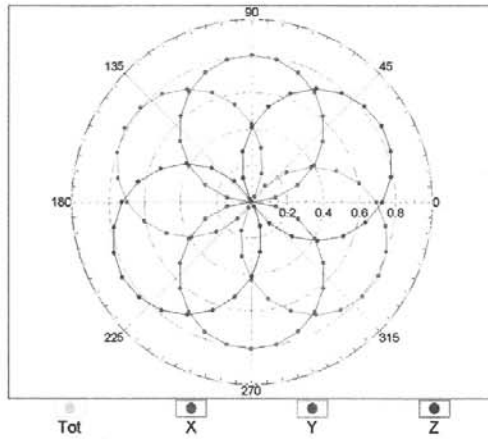
f=1800 MHz,R22
