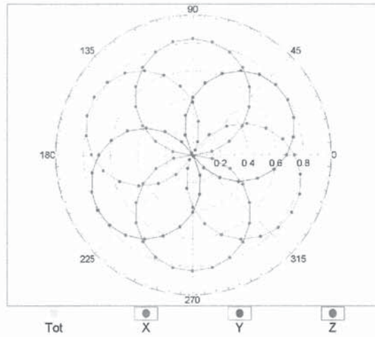
f=1800 MHz,R22
