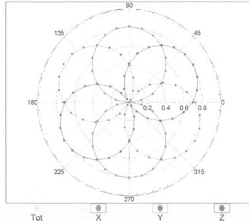
f=1800 MHz,R22
