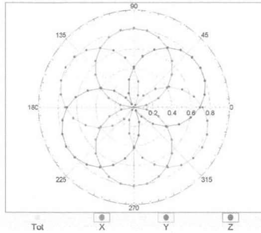
f=1800 MHz,R22
