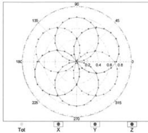
f=1800 MHz,R22
