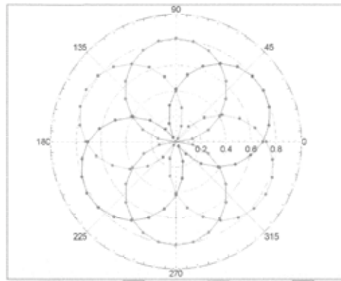
f=1800 MHz,R22
