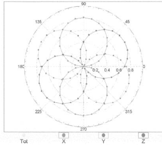
f=1800 MHz,R22
