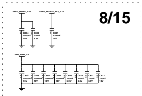
<PM IC VDD decoupling>
