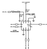
<USB_SWITCH>
