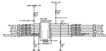
<AP & CP J-TAG >
