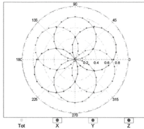
f=1800 MHz,R22
