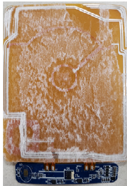
ANT Module(Back)
