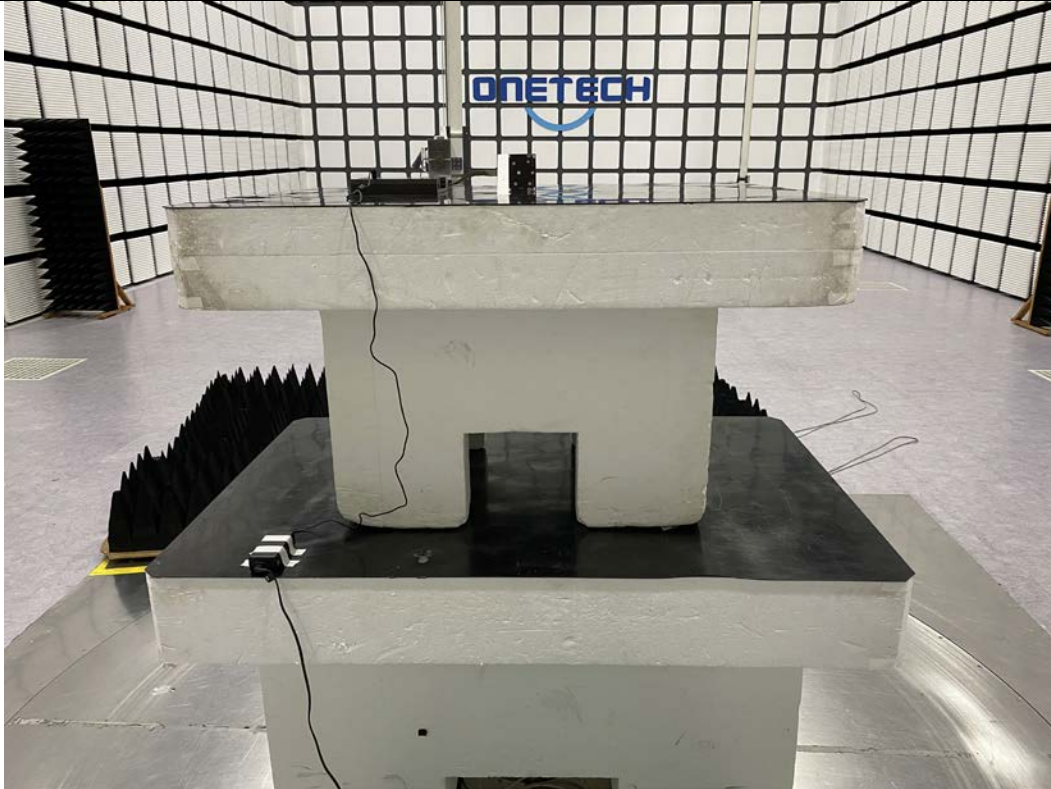
1 GHz ~ 18 GHz
