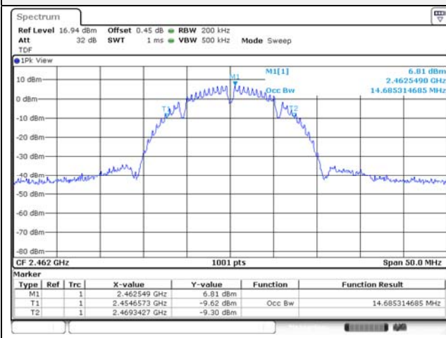
802.11b / 2 462 MHz
