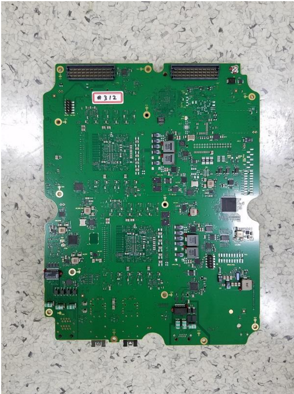
[G7DA Module_Top]
