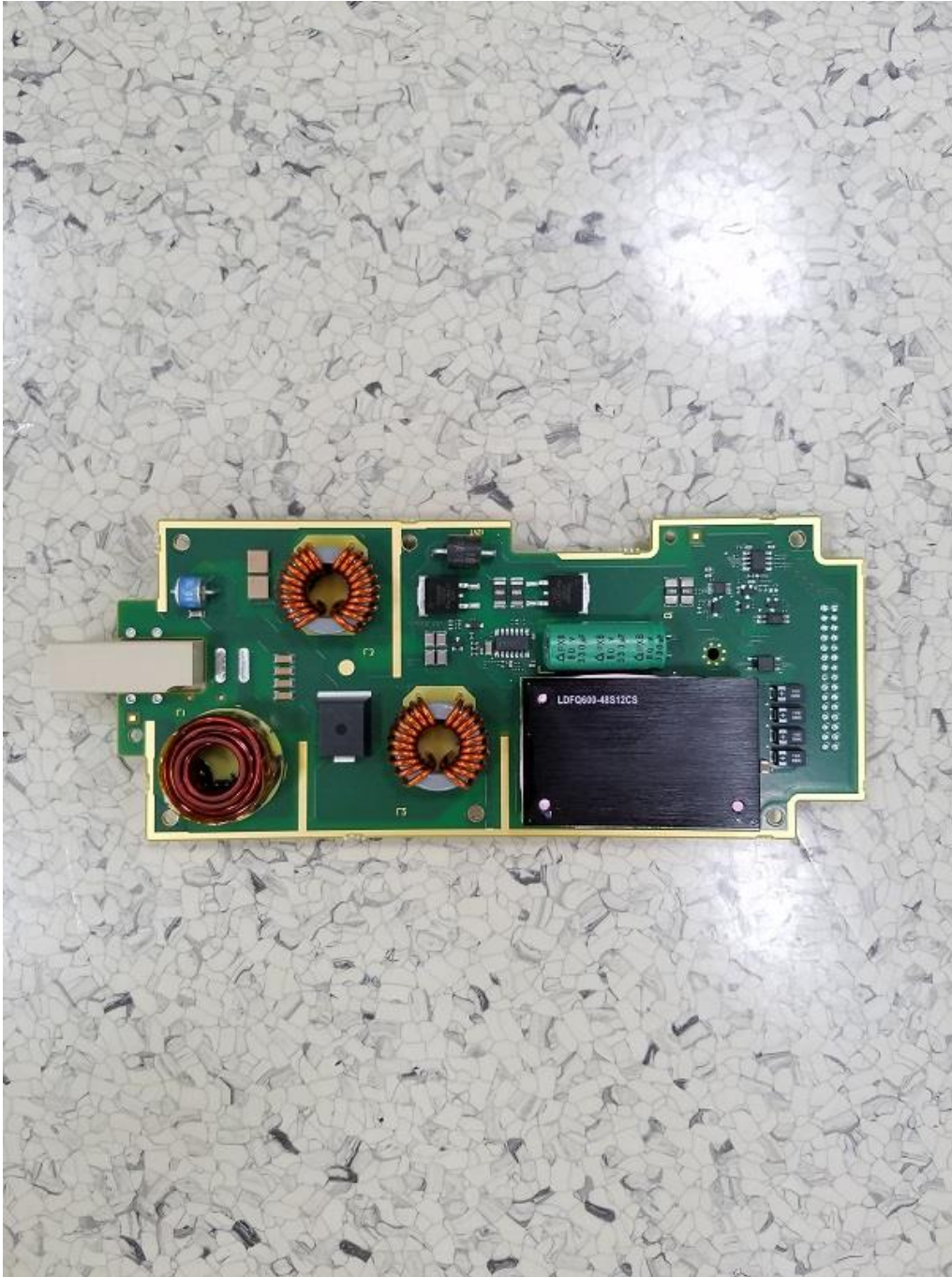
[G7PA Module_Top]
