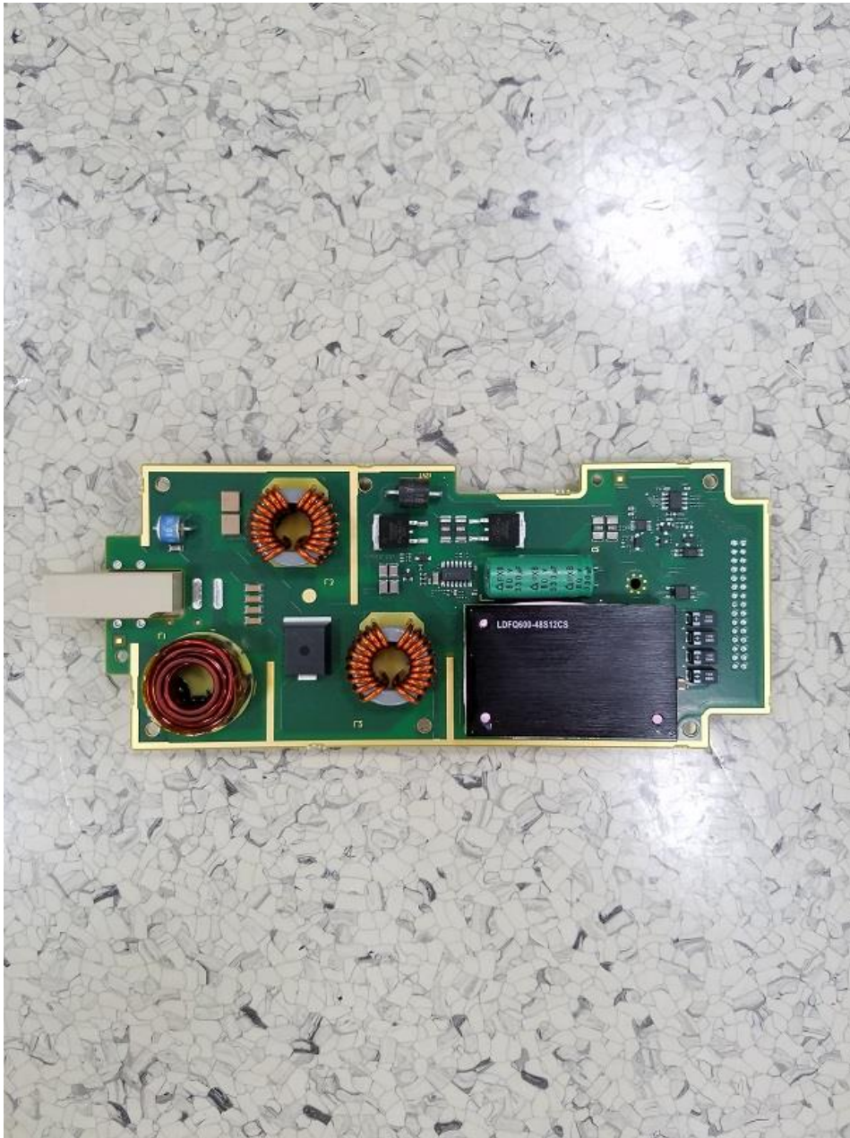
[G7PA Module_Top]
