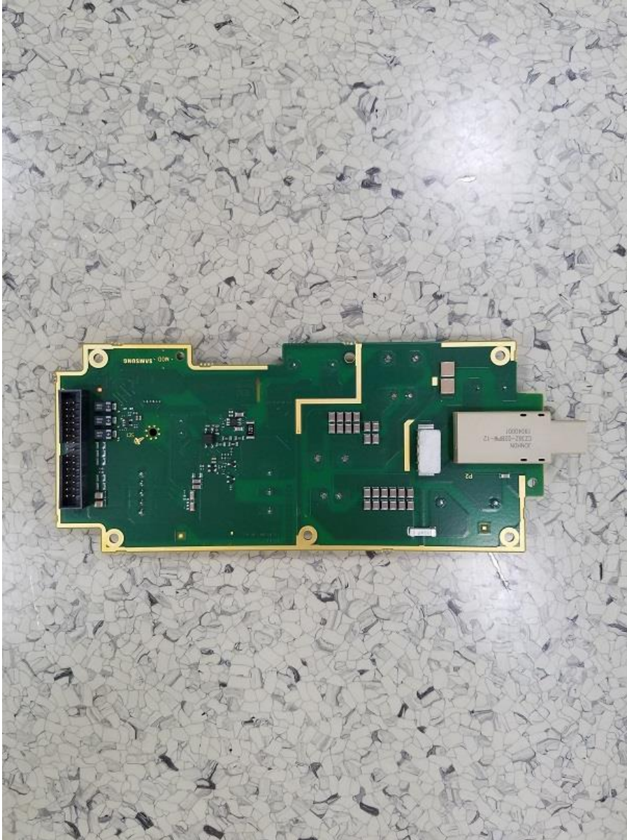
[G7PA Module_Bottom]
