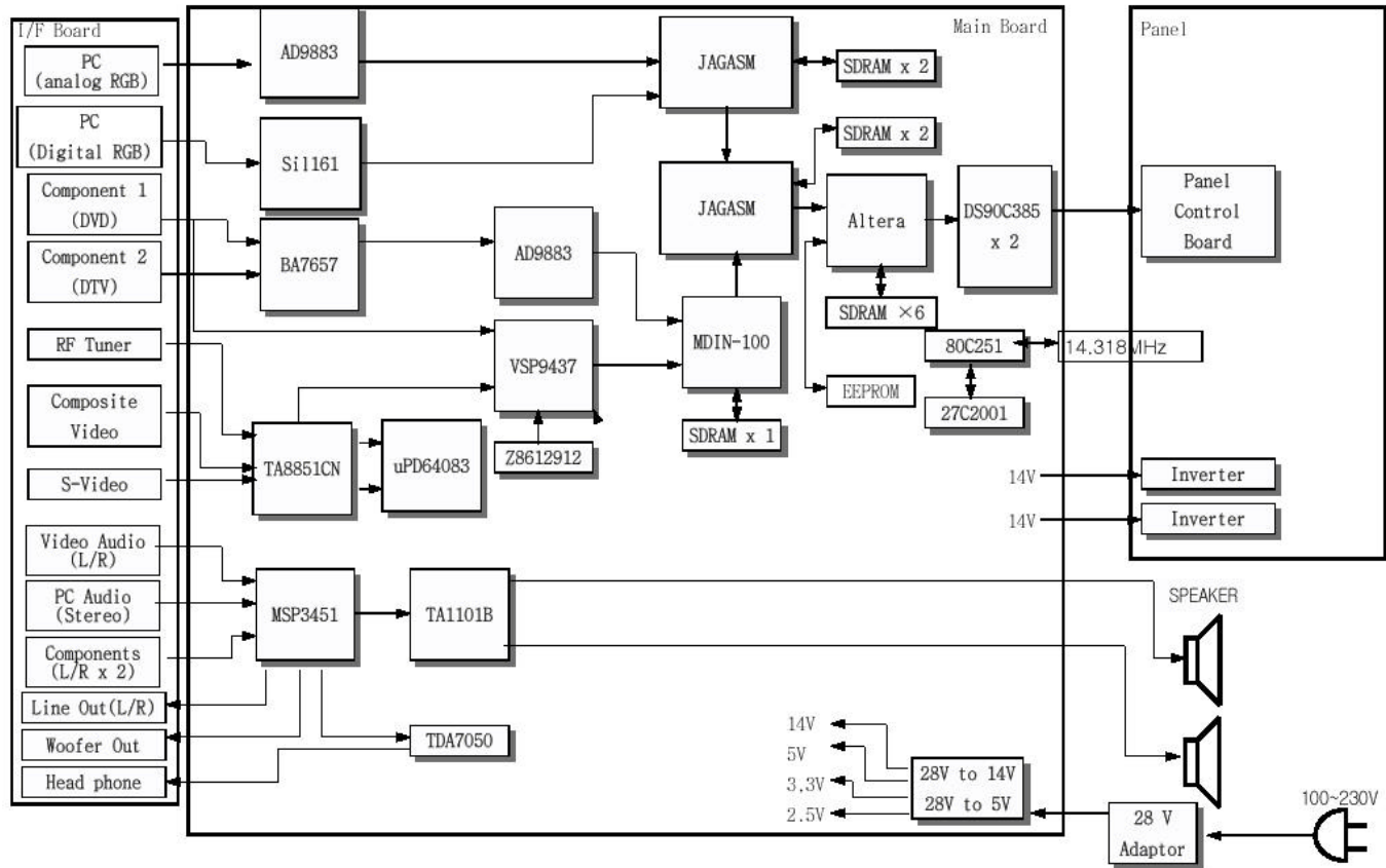
AL40NO/AN29NO Block diagram(NTSC)
