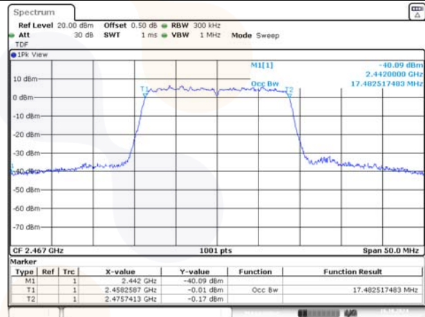
802.11n_HT20 / 2 467 MHz
