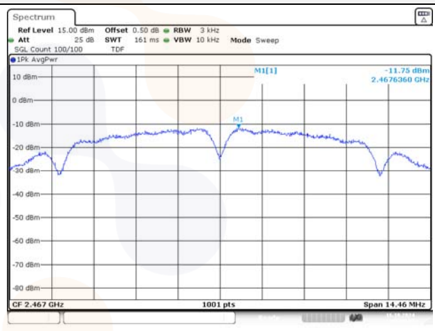
802.11b / 2 467 MHz
