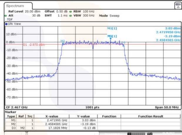
802.11n_HT20 / 2 467 MHz
