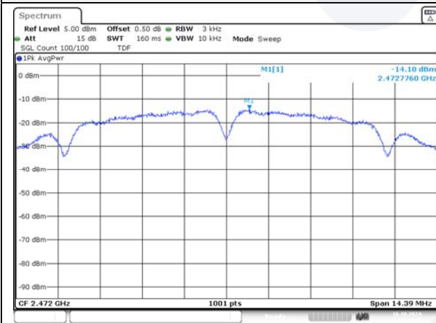
802.11b / 2 472 MHz
