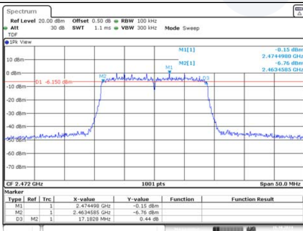
802.11n_HT20 / 2 472 MHz
