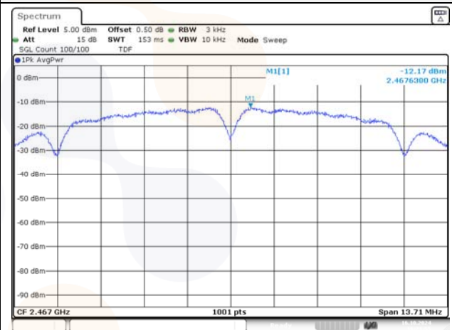
802.11b / 2 467 MHz
