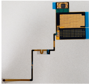
ANT Module(Back)
