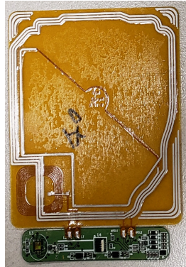
ANT Module(Back)
