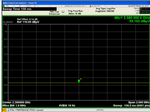
GFSK LOW FREQUENCY BAND, AV
