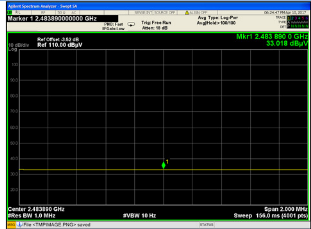
GFSK HIGH FREQUENCY BAND, AV
