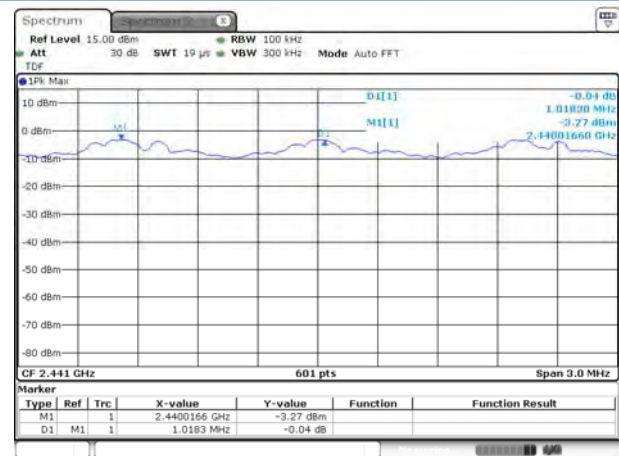
\Pi/4 -DQPSK
