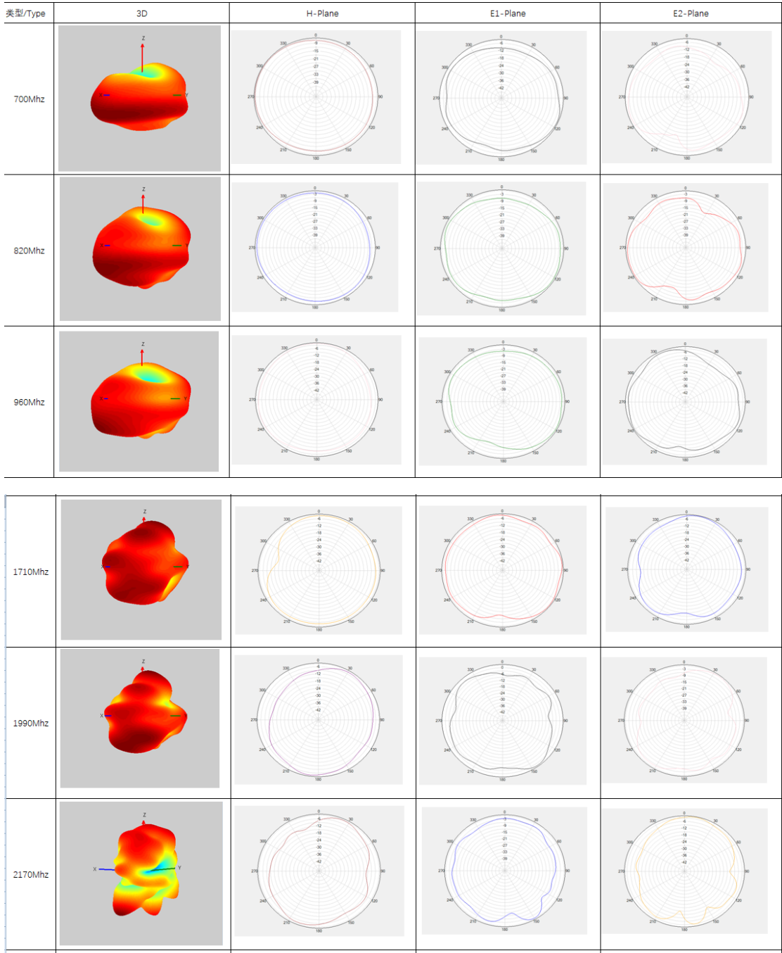
天线方向图(Antenna pattern): 主天线 Main ant
