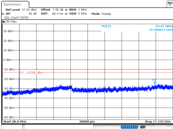
5MHz_Low_QPSK_25@0 -24.87dBm
