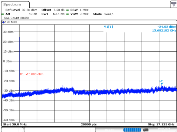
5MHz_Low_QPSK_1@0 -24.02dBm
