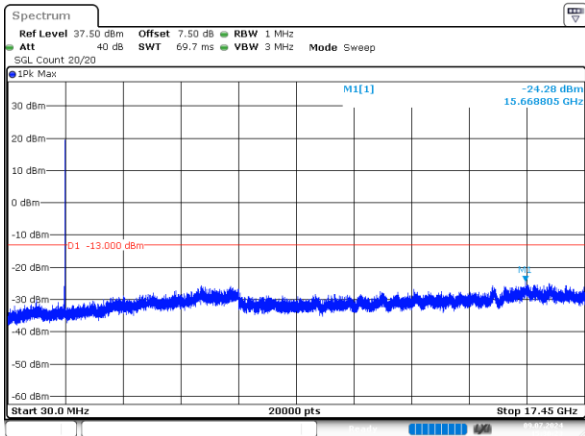
5MHz_Middle_QPSK_25@0 -24.28dBm
