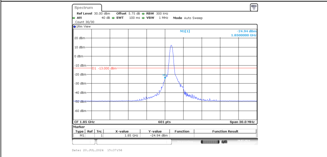
Band2-15MHz-QPSK-18675-1-0-Low--24.94-PASS
