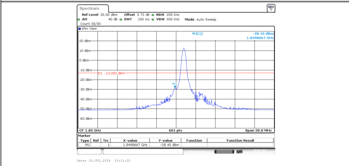
Band2-10MHz-QPSK-18650-1-0-Low--28.45-PASS
