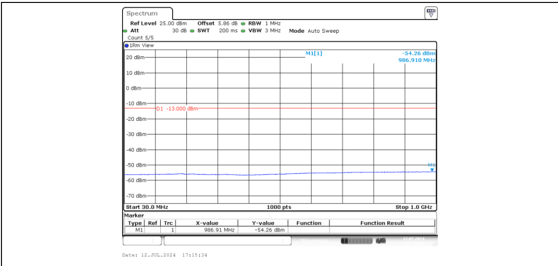
Band2-20MHz-QPSK-18900-1-0-Low-30-1000--54.26-PASS
