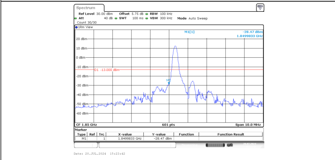
Band2-5MHz-16QAM-18625-1-0-Low--28.47-PASS
