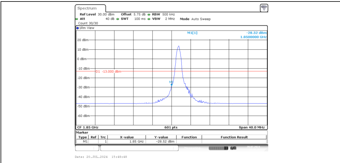
Band2-20MHz-QPSK-18700-1-0-Low--28.52-PASS
