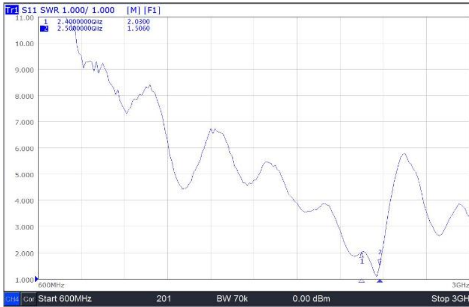
VSWR
