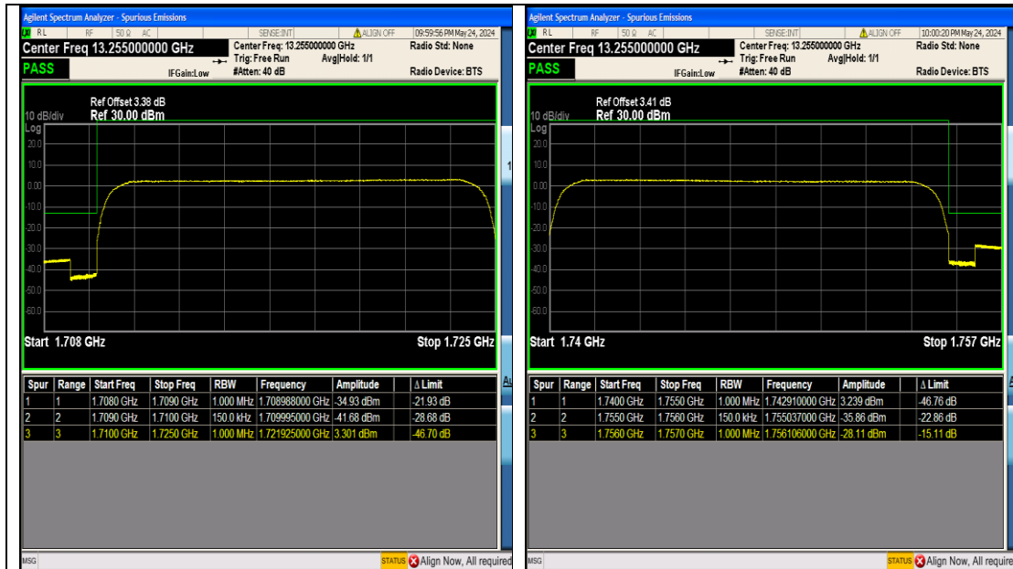
Band4_15MHz_QPSK_2025_75RB#0
