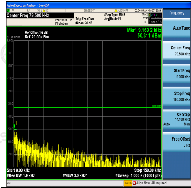
9KHz-150KHz
