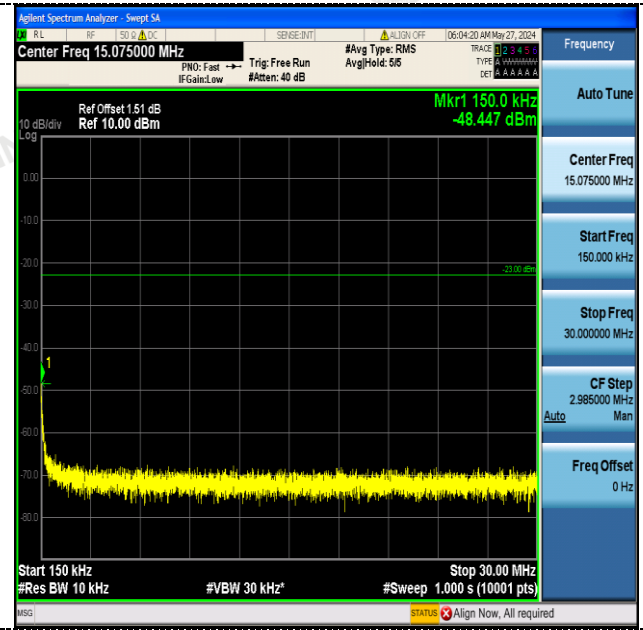
150KHz-30MHz
