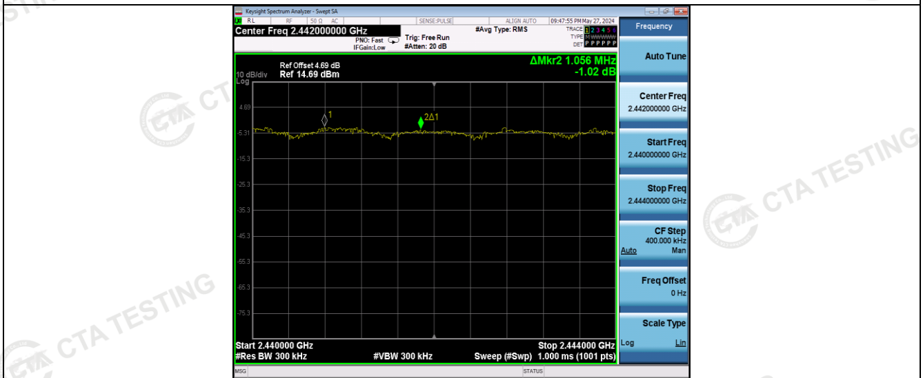
8DPSK
