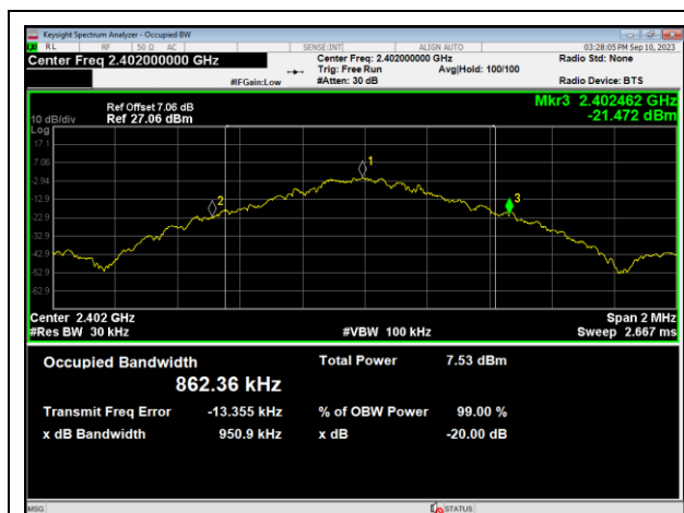
2402MHz
