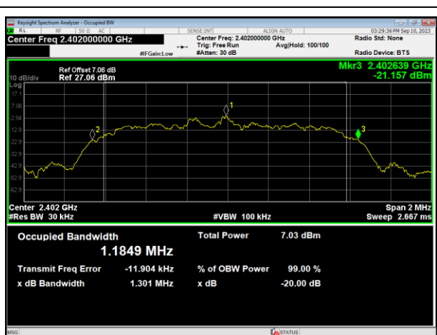
2402MHz
