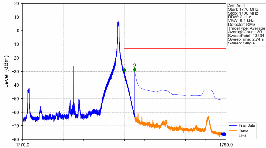
Band66_10MHz_QPSK_HCH_1775MHz_RB_1_49_NTNV
