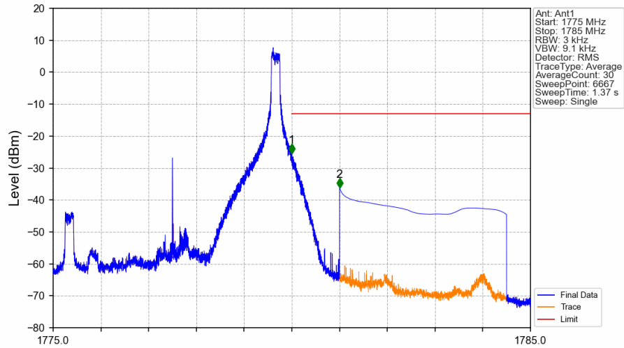
Band66_5MHz_QPSK_HCH_1777.5MHz_RB_1_24_NTNV
